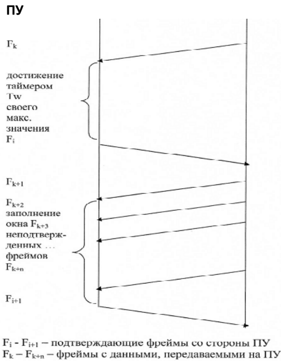
Рисунок 115. Временная диаграмма процедуры передачи.
